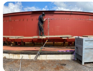
Hanover 2 storage tanks à 8,000 m 3
